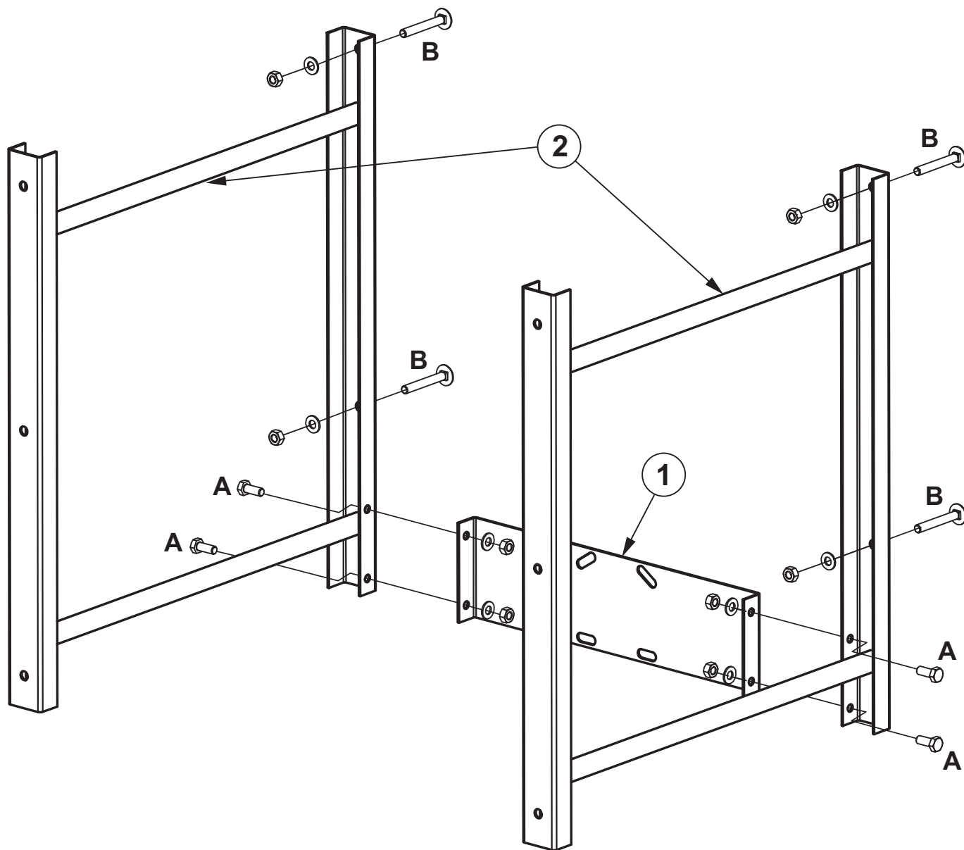
Wykaz części / Parts check list
