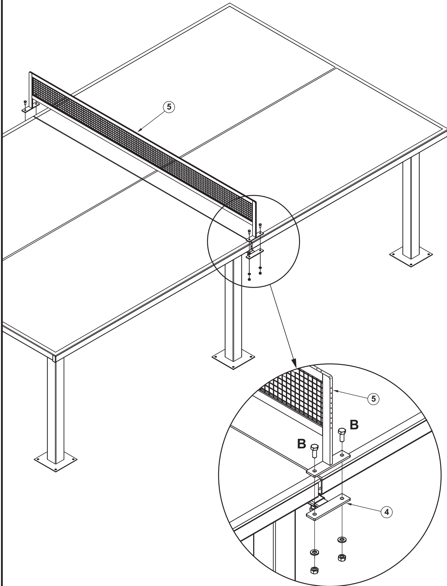
Rys. 2 / Pic 2 Montaż siatki / Legs assembly
